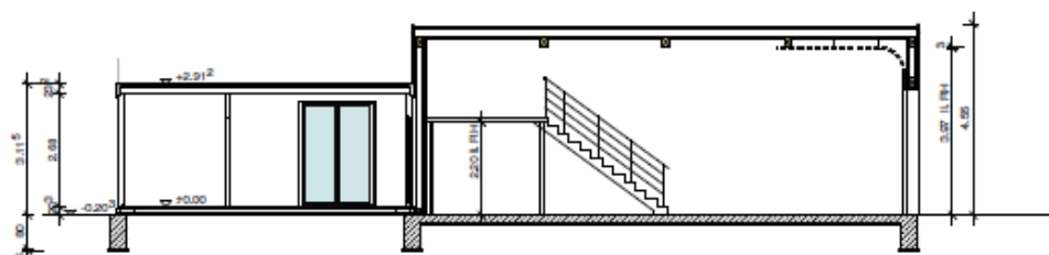
Schnitt 1-1
